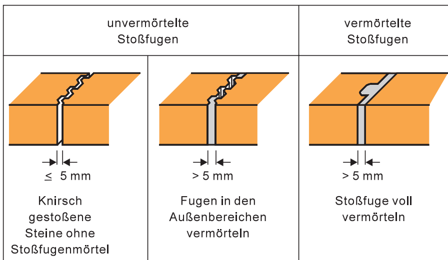
Bild 9 Stoßfugenausführung
